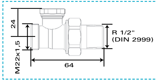
Recht M22x1,5 buitendraad
