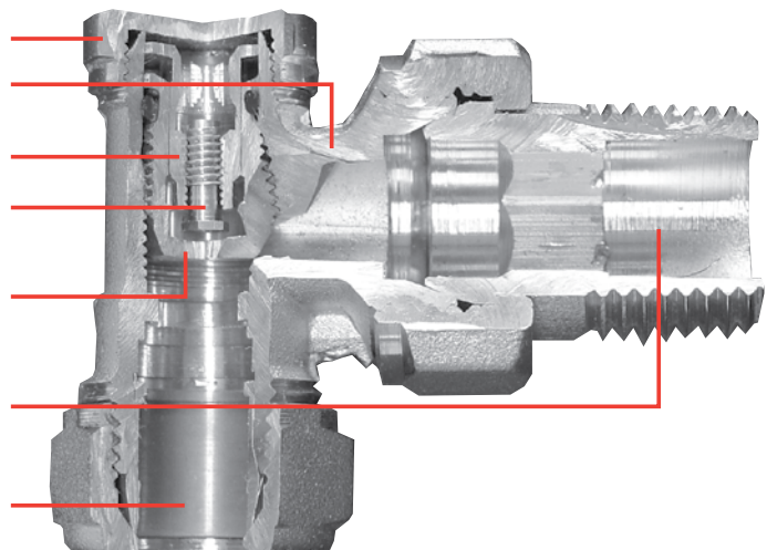
Voetventiel haaks M22 x 1,5 buitendraad
