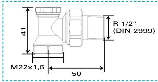
Haaks M22x1,5 buitendraad
