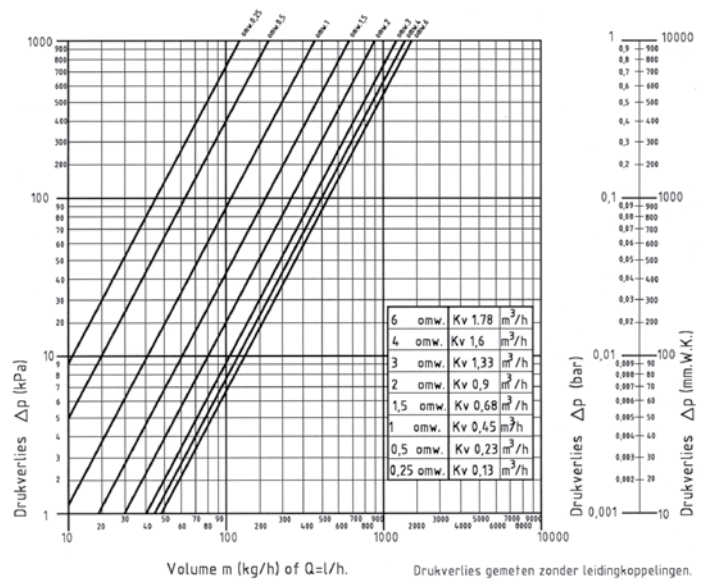
Drukverliesdiagram voetventiel recht
