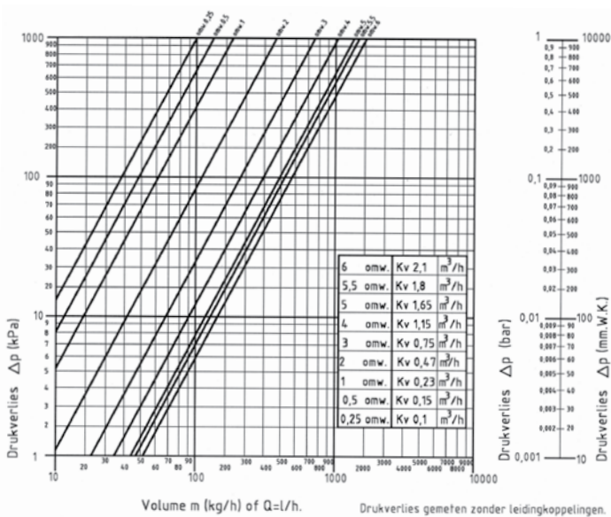
Drukverliesdiagram voetventiel haaks
