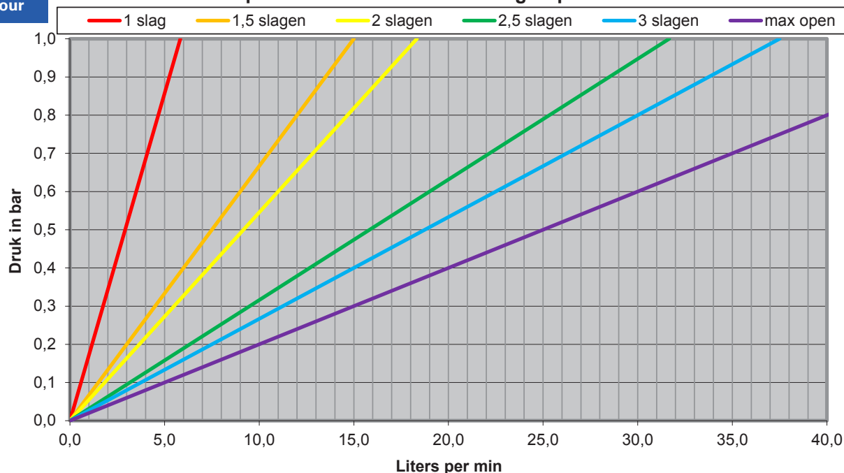
Capaciteit PenTec retourventiel-groepen Recht
