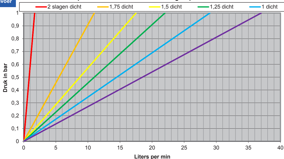
Capaciteit PenTec aanvoerventiel groepen Haaks
